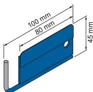
252 131 Blue - 45Ht x 100L mm
